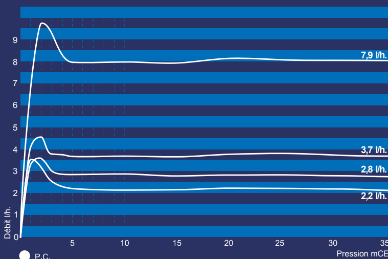
Courbes débit/pression
